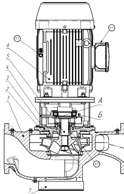
Рисунок К.1 – Электронасос центробежный консольный моноблочный типа КРЛ
