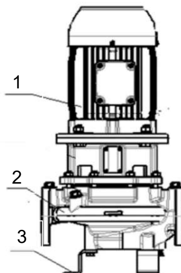
Рисунок Д.1 Схема электронасоса типа KRL на лапах. 1 – электродвигатель, 2 – блок насосный, 3 – лапка насоса.
