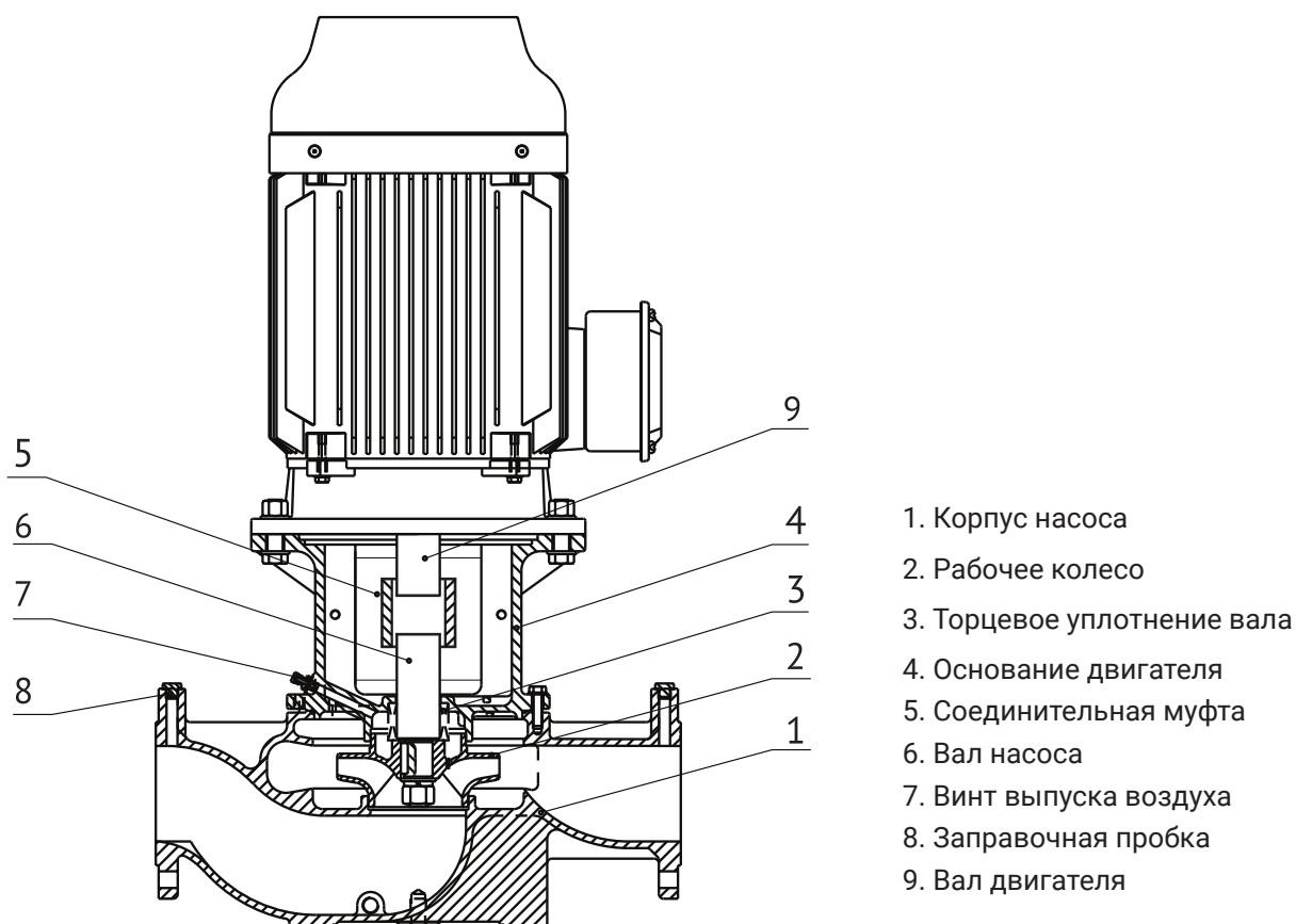
Рисунок 1. Разрез насоса TD
